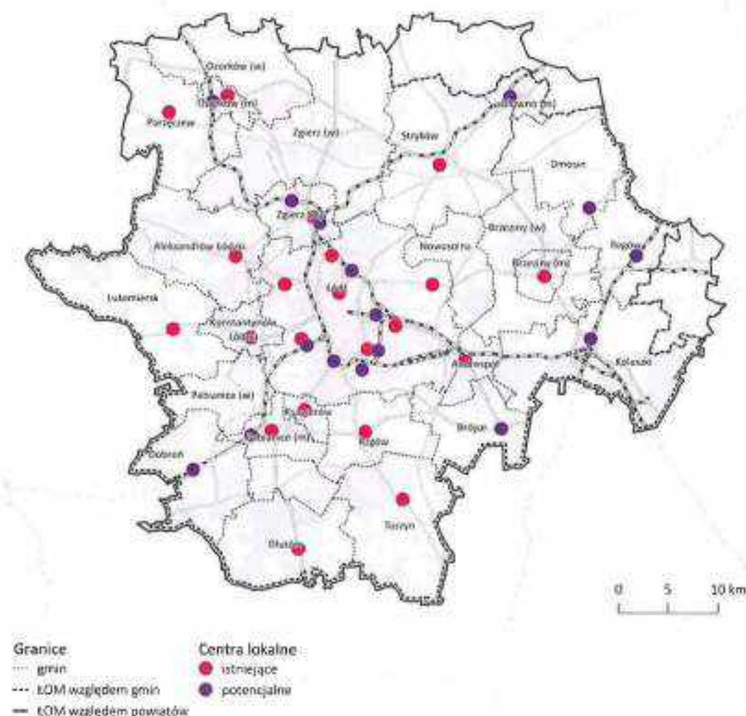
Mapa 9. Istniejące i proponowane centra lokalne na terenie ŁOM
