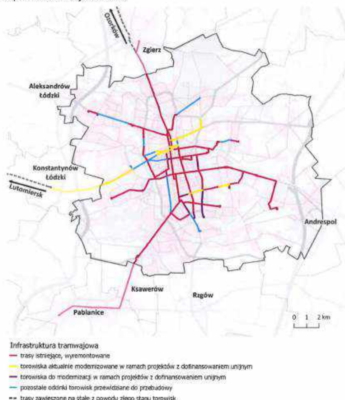
Mapa 4. Sieć tramwajowa w Łodzi
