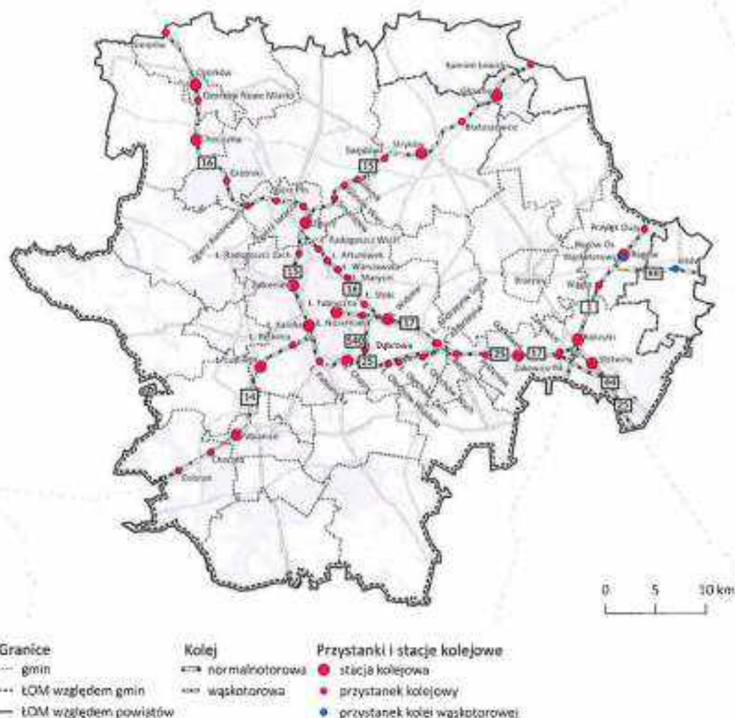
Mapa 3. Obecna sieć kolejowa na terenie ŁOM
