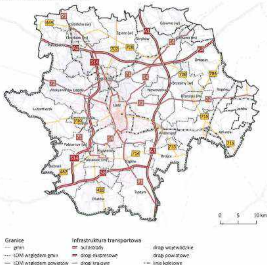
Mapa 7. Układ drogowy w ŁOM
