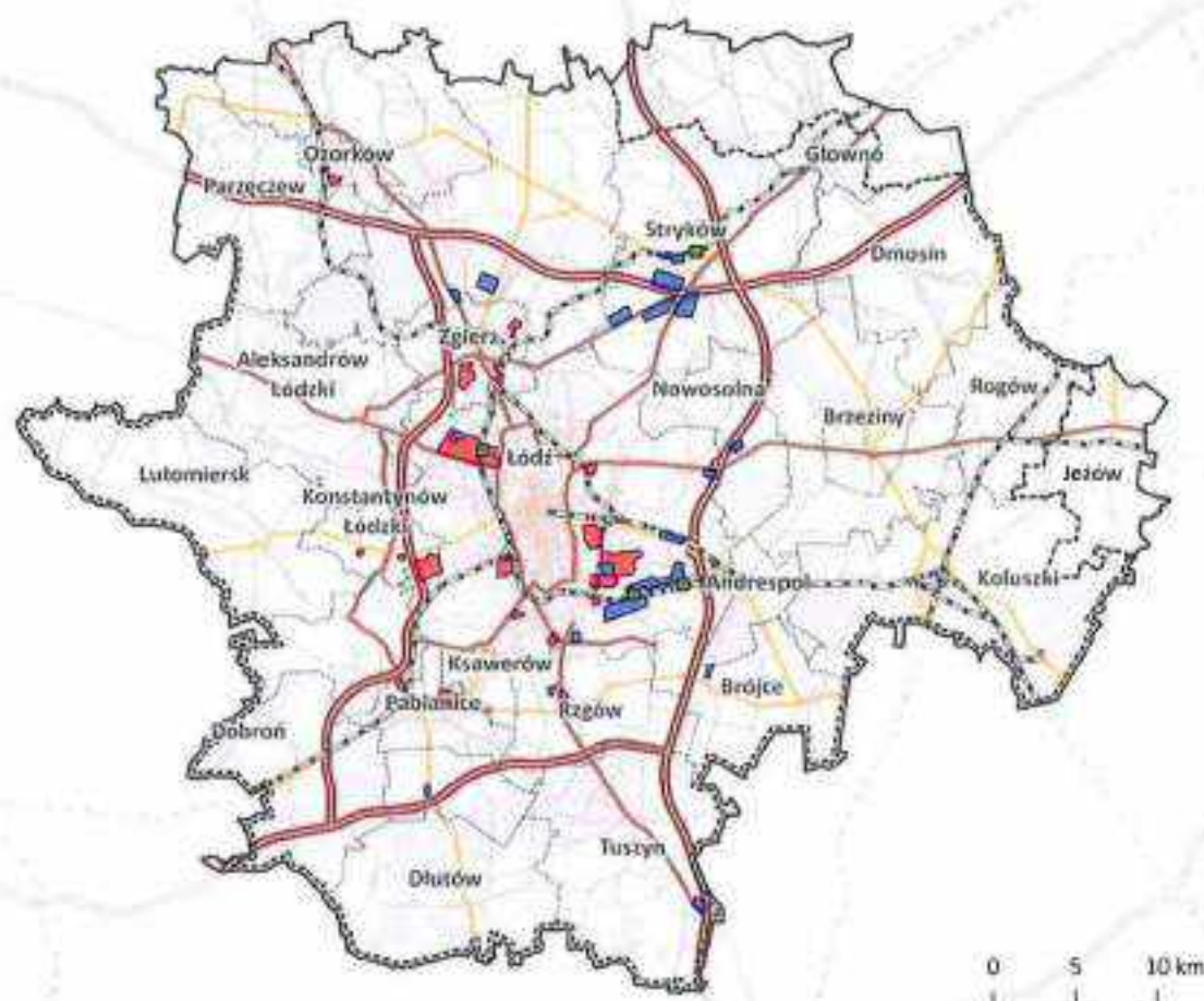
Mapa 8. Infrastruktura logistyczna w Łódzkim Obszarze Metropolitalnym
