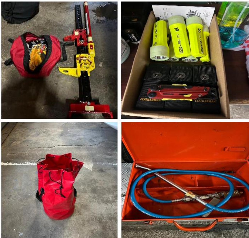
Zdjęcie 47. Podnośnik Hi-Lift, latarki oraz multitoole, sprzęt wysokościowy, lanca kominowa
