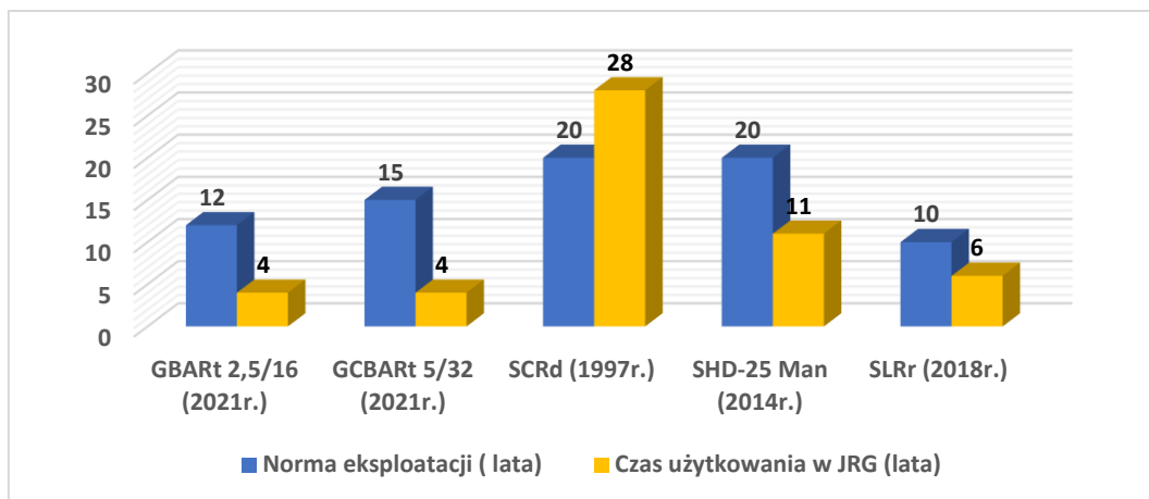
Wykres 29. Czas użytkowania pojazdów JRG Ozorków w porównaniu do normy eksploatacyjnej
