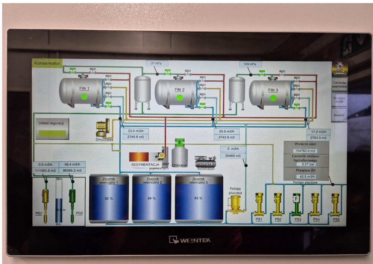
Fot. Schemat działania SUW w Strykowie
