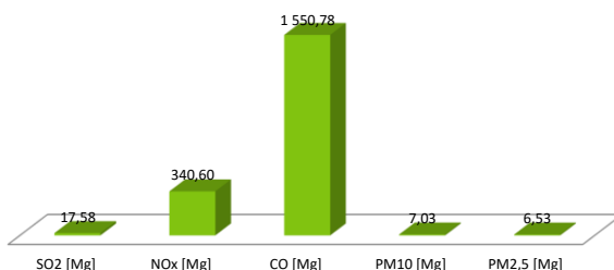
Emisja substancji szkodliwych [Mg] z transportu drogowego (samochody osobowe) na terenie Gminy Stryków w roku 2014
